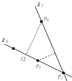
FIGURE 7.2 – La solution du problème de Sylvester par Kelly
