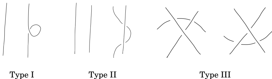
FIGURE 1.1 – Trois transformations élémentaires sur les nœuds connues sous le nom de mouvements de Reidemeister . Ces mouvements locaux transforment un diagramme de nœud en un diagramme de nœud équivalent, c'est-à-dire, représentant le même nœud.
