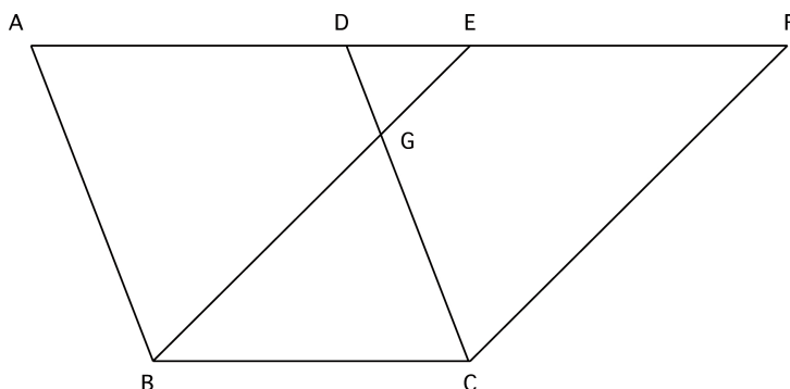
FIGURE 1.2 – Le diagramme associé à la proposition 35 du livre I des Éléments d'Euclide tel que représenté par Vitrac [Euclide d'Alexandrie, anc./1990, p. 262]. La proposition 35 énonce que « [l]es parallélogrammes qui sont sur la même base et dans les mêmes parallèles sont égaux entre eux ». Dans ce diagramme, l'égalité des segments AD et EF est un attribut exact, alors que le fait que le segment DE soit contenu dans le segment AE est un attribut co-exact. Mumma [2010, pp. 264–267] discute cet exemple de manière détaillée.
