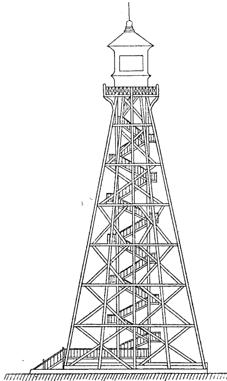
Phare en charpente de Pontailac (près de l'embouchure de la Gironde). Disposition hélicoïde de l'escalier, non isotrope autour de l'axe vertical. Paliers et rampes alternants.
