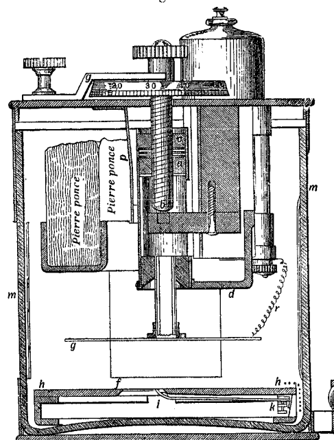
Électromètre portable, forme actuelle : \frac{2}{3} de la grandeur.
