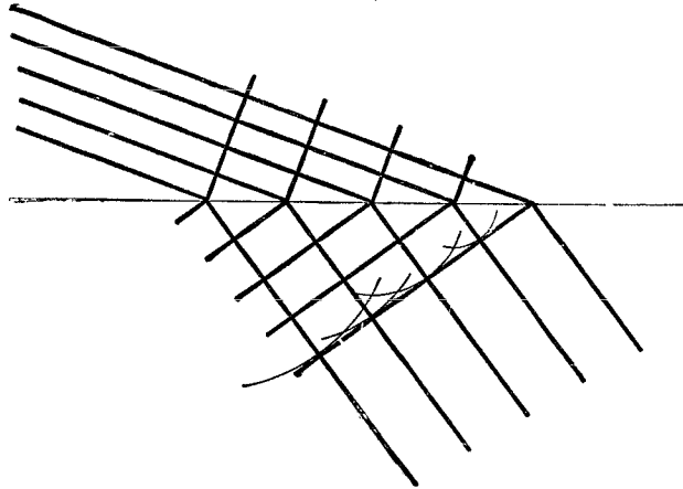
Dessin de la construction d'Huygens pour le front de l'onde réfractée; la lumière passe de l'air dans le flint-glass.
