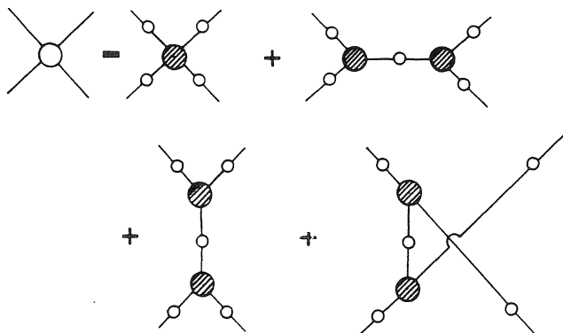
Fig. 7.2. See text.
