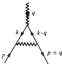
Fig. 9.7. Vertex graph.
